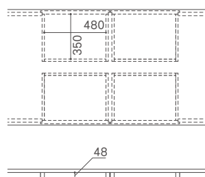
引出し内寸 (W1600-W2200)
