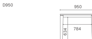
引出し内寸 (W1600-W2200)
